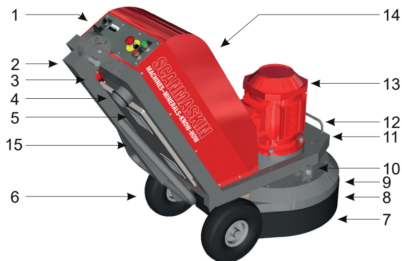
Figur 1.3 Scanmaskin 650 översikt
