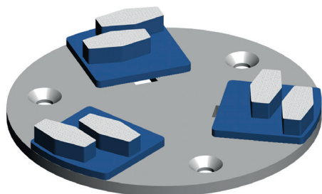
Figur 1.2 Scan-On-fästskiva med verktyg
